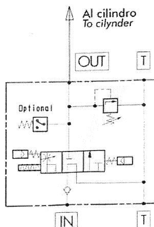
Schema di funzionamento Functional diagram
