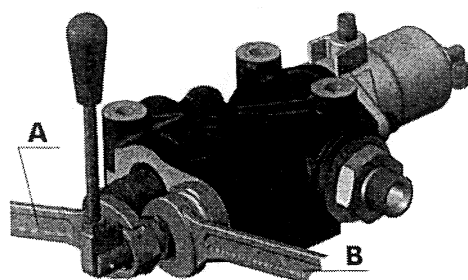
Modular con valvola doppia/tripla pressione ad azionamento meccanico. Modular with double/triple pressure valve with manual selection.
