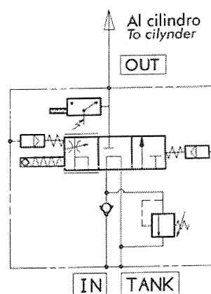
Schema di funzionamento Functional diagram
