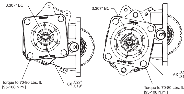
Ass'y "3"
