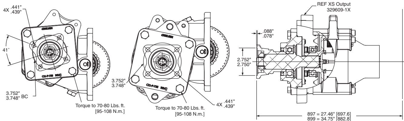
Ass'y "3"
