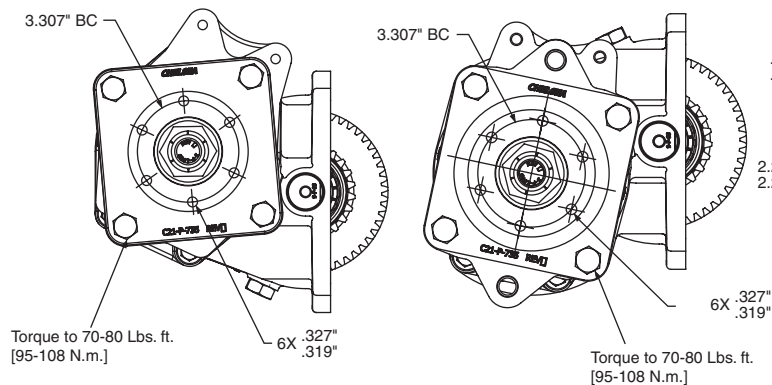
Ass'y "3"
