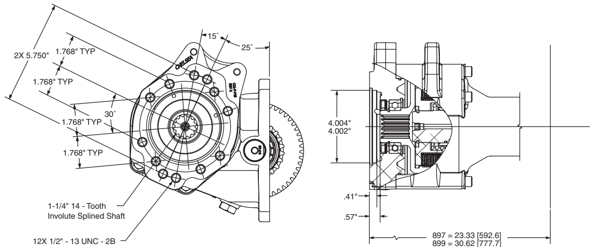
Ass'y "3"
